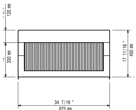
Zij aanzicht
